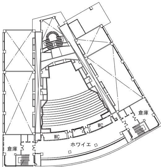
M2階
