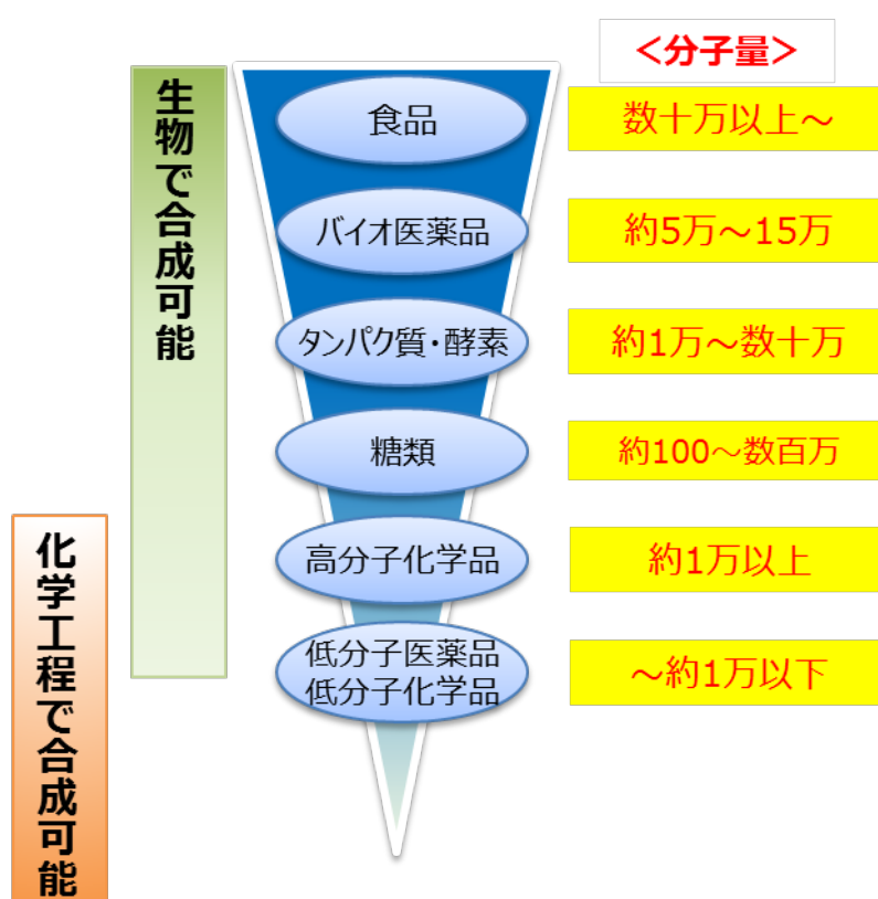
バイオ合成法と化学合成法で製造可能な化合物
