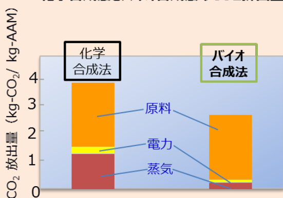
化学合成法とバイオ合成法のCO 2 排出量
