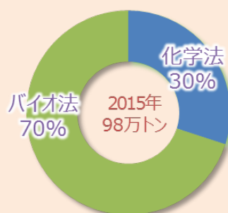
合成法別のアクリルアミドの生産割合
