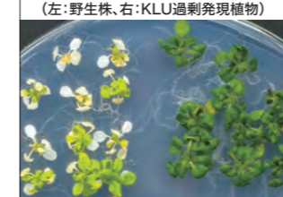
KLU遺伝子は植物の高温耐性を増強する(左:野生株、右:KLU過剰発現植物)
